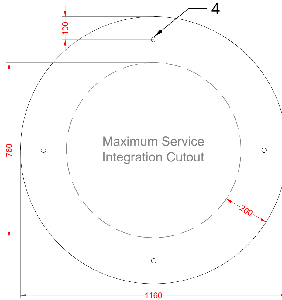
1160mm Ø Circle
